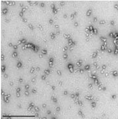
EM-Aufnahme von Amyloid-Oligomeren.
